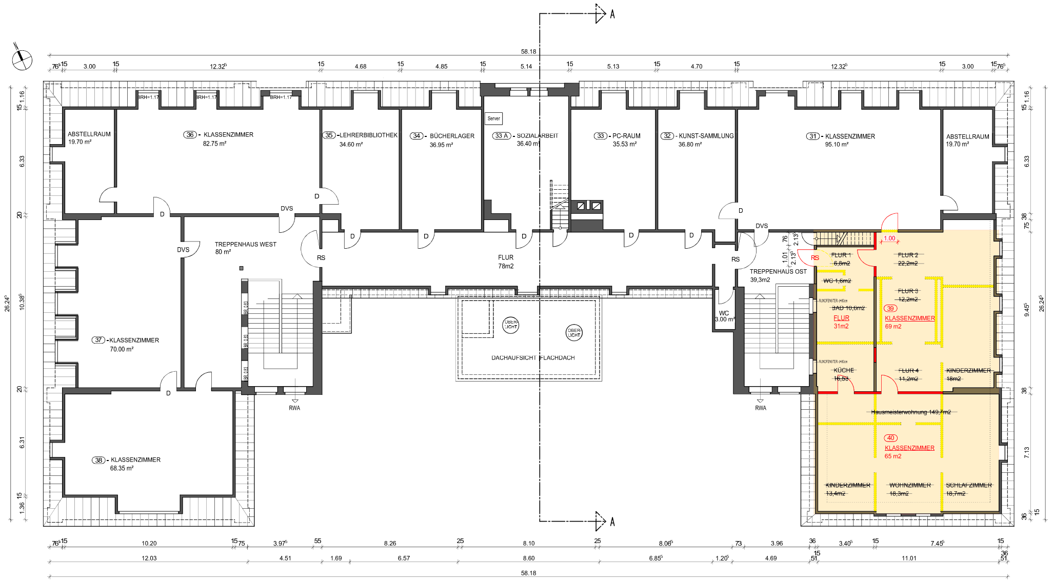
Grundriss Dachgeschoss M 1:100
